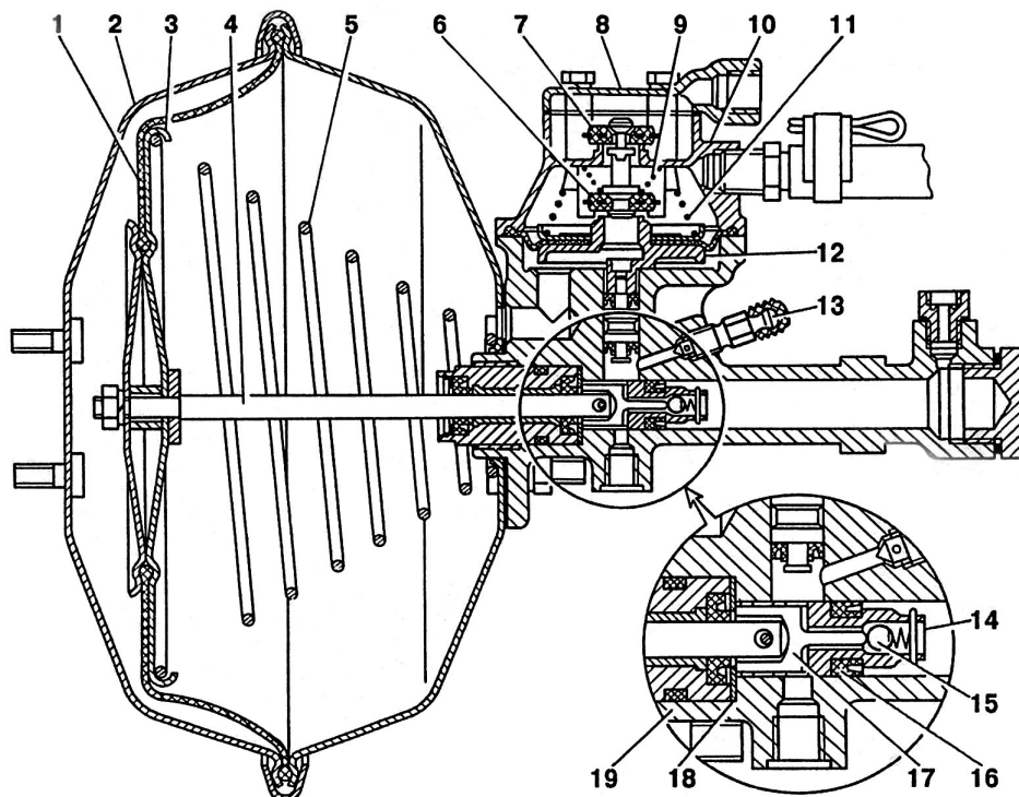
Рис. 6.18 Гидровакуумный усилитель
