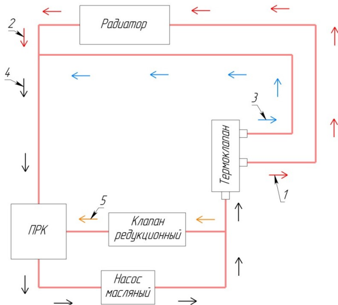
Рис. 6.5 Общая схема системы охлаждения ПРК
