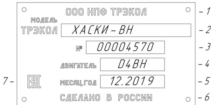
Рис. 4.2 Идентификационная табличка ВТС:
