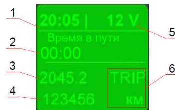
Рис. 5.19 Общий вид ЖКИ
