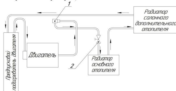
Рис. 6.21. Система отопления:
