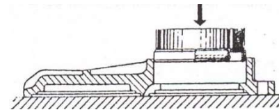
Рис.6.10 Запрессовка манжеты
