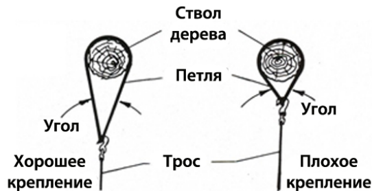
Рис. 19.7 Петля.
