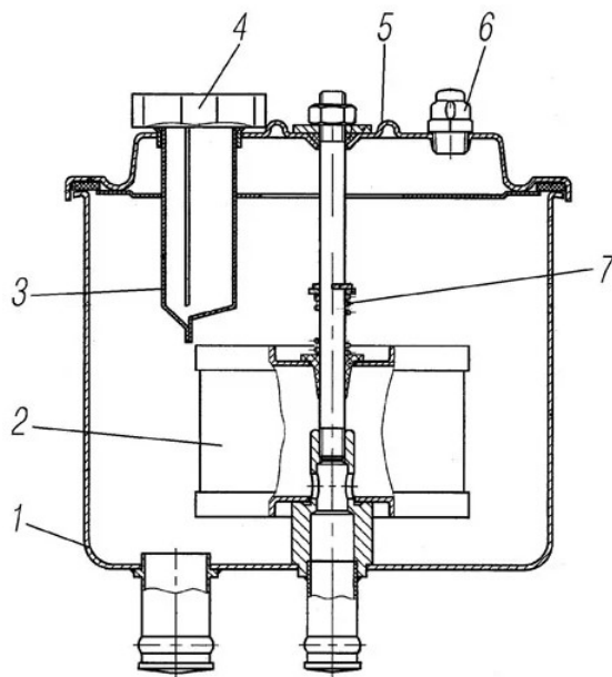
Рис. 6.14 Бачок усилителя рулевого управления:
